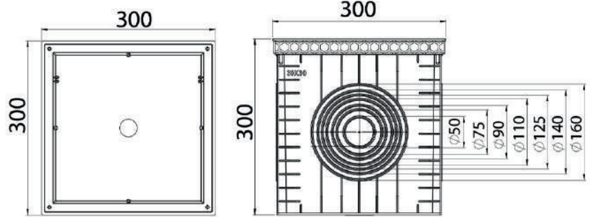
30x30 CM YÜKSEKLİK/HEIGHT 300 MM
