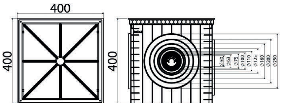
40x40 CM YÜKSEKLİK/HEIGHT 400 MM
