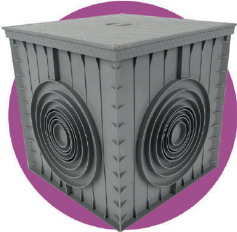
35x35 CM YÜKSEKLİK/HEIGHT 350 MM
